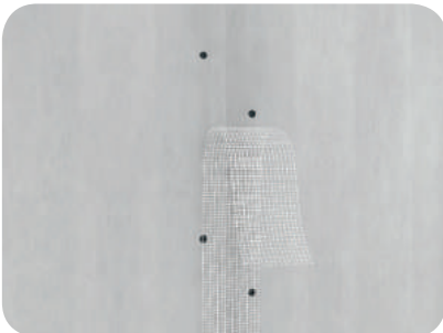
Рис. 7.16. Приклеювання стрічки зі скловолна на стики плит
