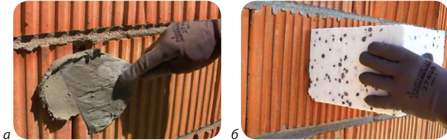
Рис. 9.7. Пробне приклеювання пінополістиролу: а – нанесення клейового розчину; б – притискання зразка пінополістиролу
