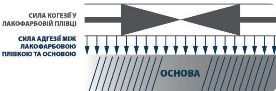
Рис. 2.6. Адгезія і когезія в лакофарбовій плівці
