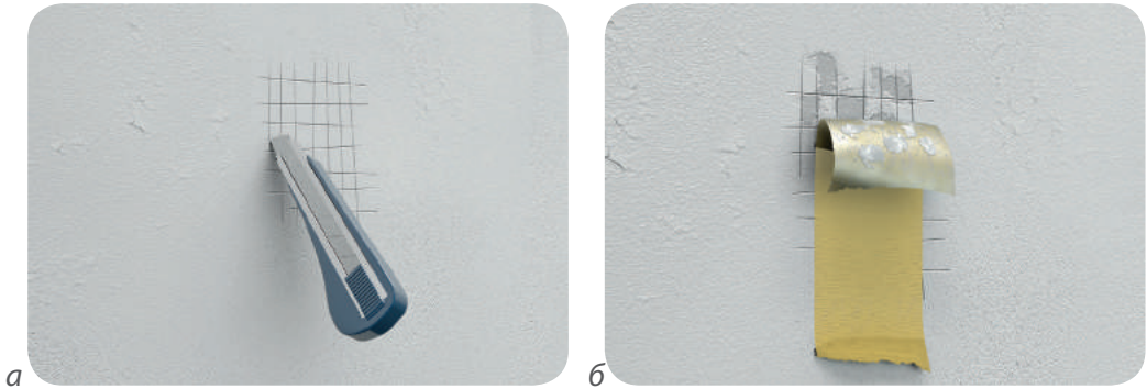
Рис. 7.6. Перевірка адгезії старого покриття методом «сітчастих надрізів»: а – виконання надрізів; б – відривання малярної стрічки
